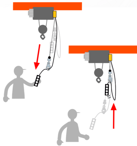
天井クレーンの ペンダントのけんすい
